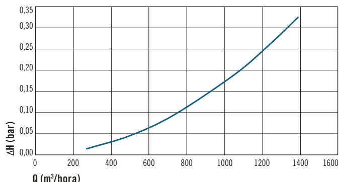
Válvulas / Valves DN 300
