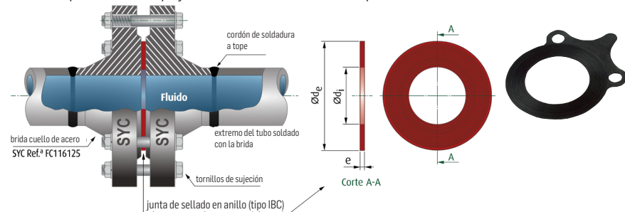
Figura 11 Junta de sellado con cara total UNE-EN 1514-1 (tipo FF) - Aplicada a un par de Bridas SYC Ref.ª FC016125, planas para soldar y cara plana: EN 1092-1 - Tipo 01 - Cara A - DN 125 - PN 16 - P245GH
